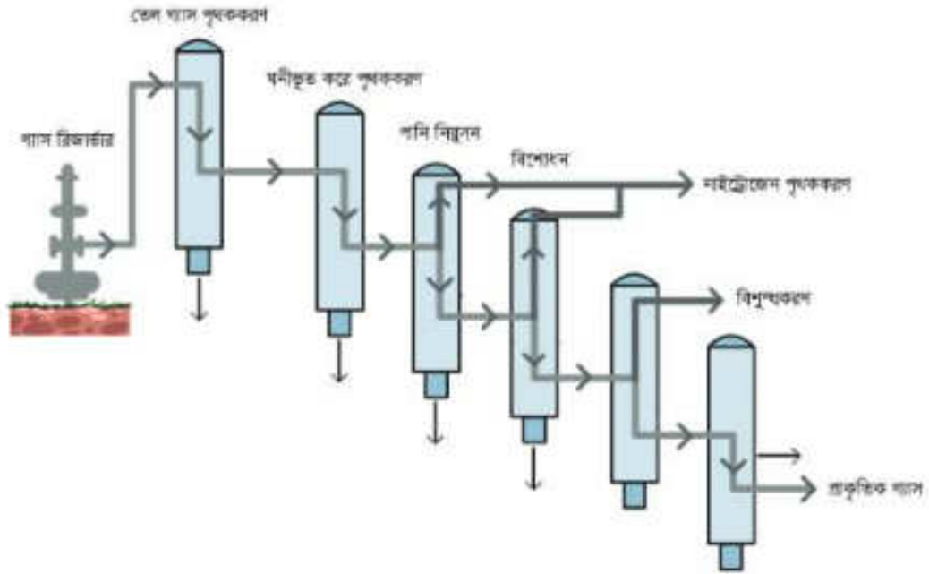
চিত্র ৮.০৩: প্রাকৃতিক গ্যাস প্রক্রিয়াকরণ
