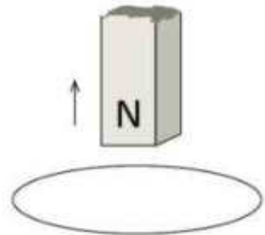
চিত্র 12.14: একটি লুপের ভেতর একটি চুম্বকের অবস্থানের পরিবর্তন।
