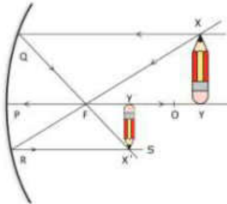
চিত্র 8.24: অবতল আয়নার একটি বস্তু ফোকাস দূরত্বের দ্বিগুণ দূরত্বের বাইরে রাখলে প্রতিবিম্বটি উল্টো এবং ছোট হয়।
