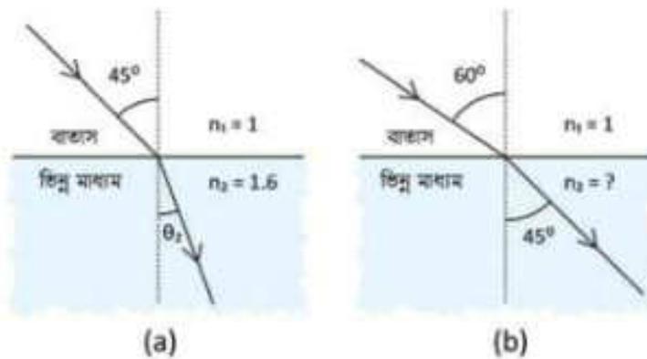
চিত্র ৯.০৪: (a) আলো 45^\circ কোণে আপতিত হচ্ছে (b) আলো 60^\circ কোণে আপতিত হয়ে 45^\circ কোণে প্রতিসরিত হচ্ছে।
