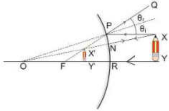
চিত্র 8.19: উত্তল আয়নার একটি বস্তু XY ফোকাস নুরের ভেতরে রাখা হলে প্রতিবিম্ব X'Y' ছোট দেখায়।
