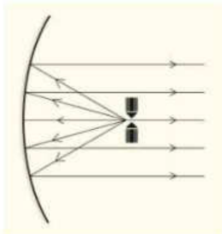
চিত্র 8.27 ফোকাস দূরত্বে তীব্র আলো তৈরি করতে সেটি অবতল আয়নায় প্রতিফলিত হয়ে সমান্তরাল আলো হিসেবে বের হয়ে আসবে।
