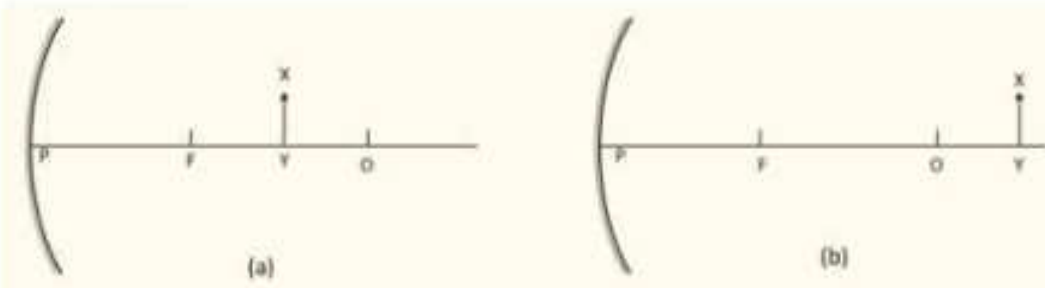
চিত্র ৪.৩০: (a) অবতল আয়নার ফোকাস দূরত্বের বাইরে রাখা একটি বস্তু। (b) অবতল আয়নার দ্বিগুণ ফোকাস দূরত্বের বাইরে রাখা একটি বস্তু।
