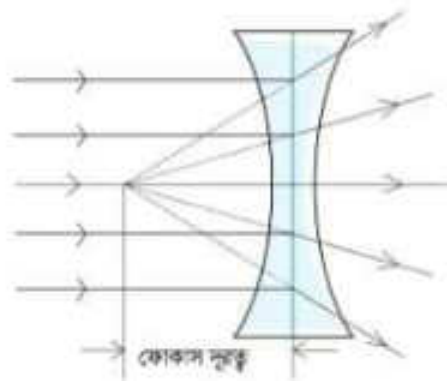
চিত্র 9.18: অবতল লেন্সের ক্ষেত্রে দিয়ে হওয়ার সময় সমান্তরাল রশ্মি ছড়িয়ে পড়ে।
