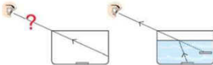
চিত্র 9.03: পানি ও কাঁচের ভেতর আলোর প্রতিসরণ।
