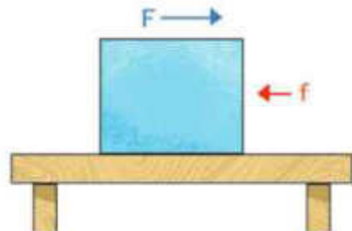
চিত্র 3.15: একটি সরের উপর বল প্রয়োগ করলে ঘর্ষণের জন্যে বিপরীত দিকে একটি বল তৈরি হতে পারে।
