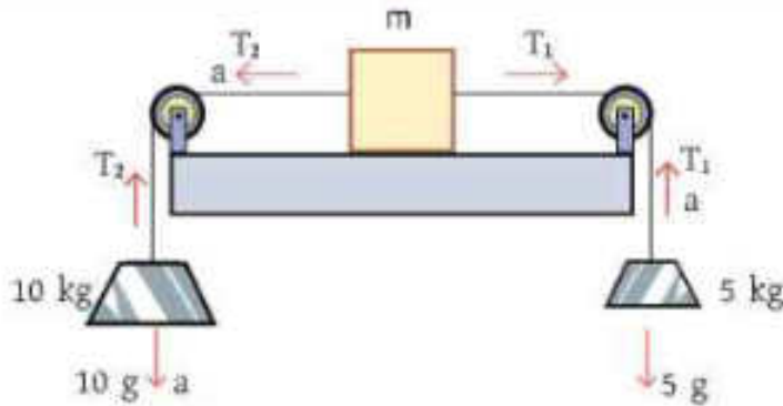
চিত্র 3.10: কণিকার দ্বারা একটি ভরকে দুই পাশে থেকে দুটি বস্তুনের মাধ্যমে বল প্রয়োগ করা হচ্ছে
