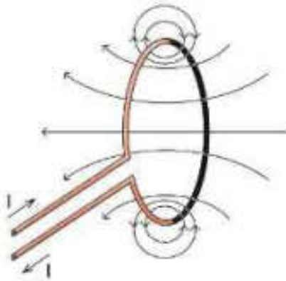
চিত্র 12.05: লুপের ভেতর দিয়ে বিদ্যুৎপ্রবাহের কারণে তৈরি চৌম্বক ক্ষেত্র।
