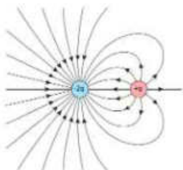
চিত্র 10.13: চার্জ এবং দ্বিগুণ পরিমাণ বিপরীত চার্জের জন্য বলরেখা।
