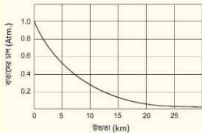
চিত্র ৫.০৭: উচ্চতার সাথে বাতাসের চাপ কমে যায়
