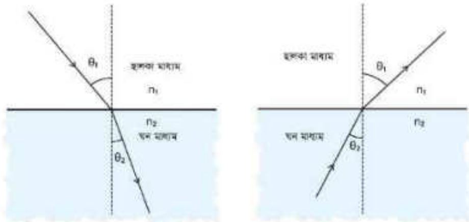
চিত্র 9.02: হালকা মাধ্যম থেকে ঘন মাধ্যমে ইওরার সময় আলো লম্বের দিকে বেঁকে যায়। ঘন মাধ্যম থেকে হালকা মাধ্যমে যাবার সময় আলো লম্ব থেকে দূরে সরে যায়।
