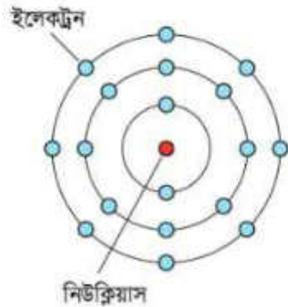
চিত্র 10.01: একটি আয়নিত পরমাণুর মডেল। এক কক্ষপথ পূর্ণ করে ইলেকট্রন পরের কক্ষপথে যায়।
