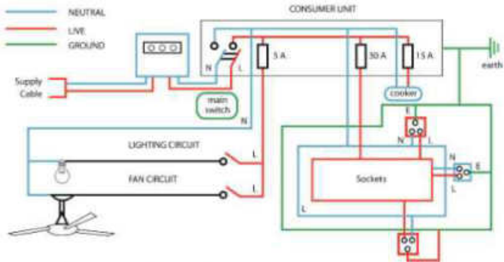
চিত্র 11.17: একটি বাসায় বিদ্যুৎ সরবরাহ করার জন্য সম্ভাব্য বিদ্যুৎ বণ্টনী।
