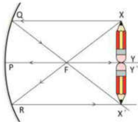
চিত্র ৪.২৫: অবতল আয়নার ফোকাস দূরত্ব এর দ্বিগুণ দূরত্বে একটি বস্তু রাখলে প্রতিবিম্বটি ঠিক একই জায়গায় উল্টো অবস্থায় দেখা যায়।
