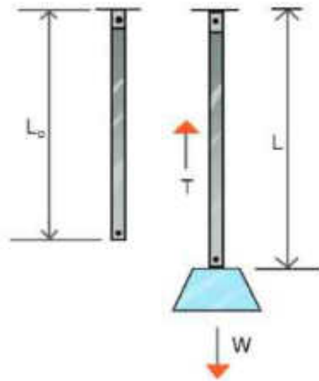
চিত্র 5.11: বল প্রয়োগ করলে দড়ের বিকৃতি ঘটে এবং সে জন্য পীড়ন সৃষ্টি হয়।
