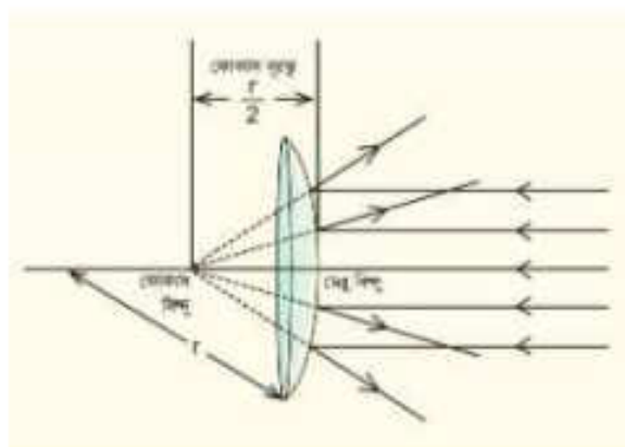
চিত্র ৪.১৭: উত্তল আয়নার ফোকাস দূরত্ব গোলকের ব্যাসার্ধের অর্ধেক।
