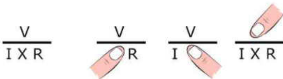
চিত্র 11.05: এ'মের সূত্র এই চিত্রটি দিয়ে ব্যবহার করা সম্ভব। আঙুল দিয়ে ঢাকা রাশিটির মান বাকি দুটি রাশি দিয়ে প্রকাশ করা সম্ভব।
