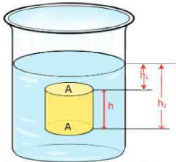
চিত্র 5.04: একটি কতু যতটুকু তরল অপসারিত করে তার সমপরিমাণ ওজন হারায়।
