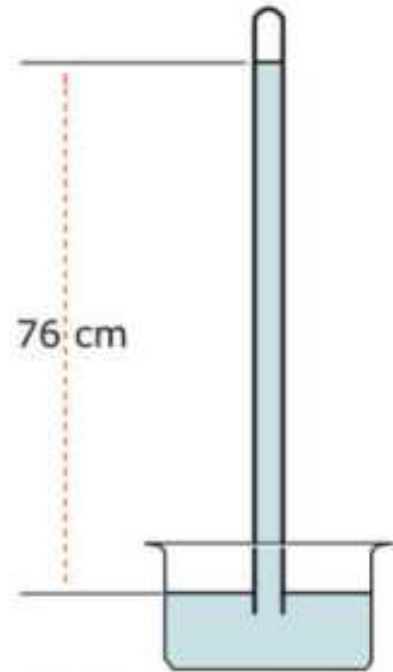
চিত্র 5.10: বাতাসের চাপের কারণে পারদ ঠিক ৭৬ cm উচ্চতায় পিঁথর হয়ে যায়।
