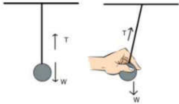
চিত্র 3.02: প্রথম ছবিতে বলের একটি সাম্যাবস্থা আছে। দ্বিতীয় ছবিতে পেঁচুলামটি ছেড়ে দেওয়া মাত্র একটি লব্ধি বল কাজ করবে, যে কারণে পেঁচুলামটি দুলতে শুরু করবে।
