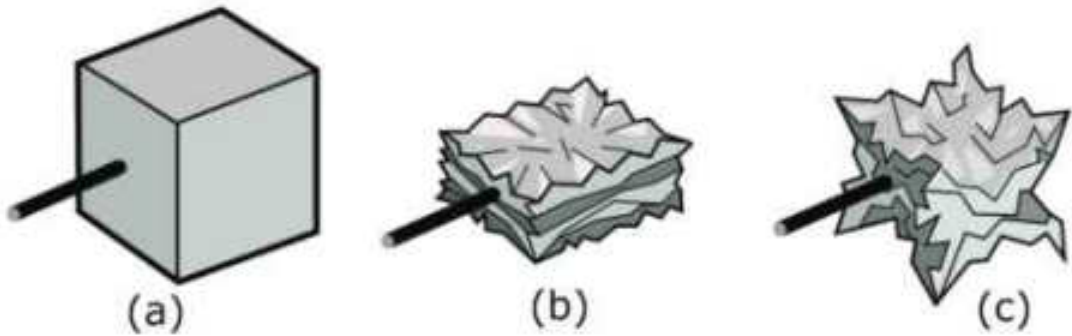
চিত্র 5.07: (a) কে দেখানো কিউবটির ভেতর থেকে পাশ করি বাতাস সরিয়ে নিলে যদি শুধু উপর থেকে চাপ দিত তাহলে (b) ছবির মতো চ্যাপ্টা হয়ে যেত। কিন্তু যেহেতু চারদিক থেকে চাপ আসে তাই (c) ছবির মতো সংকুচিত হয়।
