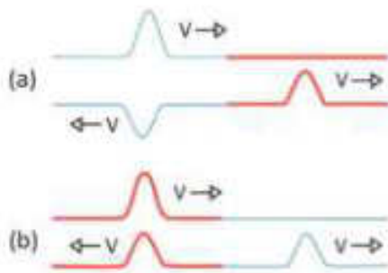
চিত্র 7.02: ভিন্ন প্রস্থচ্ছেদের তরঙ্গের তেজের একটি তরঙ্গ প্রতিফলিত এবং প্রতিসরিত হচ্ছে। (a) সরু তার থেকে মোটা তারে গেলে এক ধরনের প্রতিফলন হয় আবার (b) মোটা তার থেকে সরু তারে গেলে অন্য ধরনের প্রতিফলন হয়।
