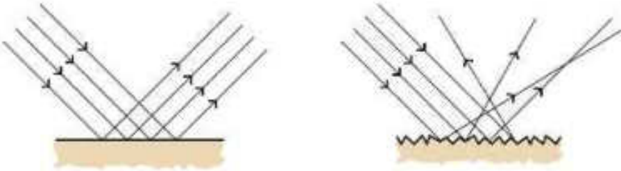
চিত্র 8.07: মসৃণ পৃষ্ঠে আলো প্রতিফলিত হয় কিন্তু অমসৃণ পৃষ্ঠে আলো বিজ্ঞুরিত হয়।
