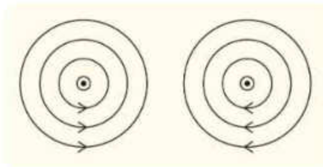
চিত্র 12.04: বিদ্যুৎপ্রবাহী তারকে ঘিরে চৌম্বক ক্ষেত্র। কোনটি সঠিক?
