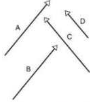
চিত্র 2.03: A ও B ভেক্টর দুইটি এক, যদিও ভিন্ন অবস্থানে রয়েছে, C ভেক্টর A ও B থেকে ভিন্ন, কারণ মান সমান হলেও দিক ভিন্ন। D ভেক্টর C ভেক্টর থেকে ভিন্ন, কারণ দিক একই হলেও মান সমান নয়।
