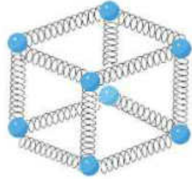
চিত্র 6.03: অণুগুলো একটি অন্যটির সাথে স্থিৎ দিয়ে যুক্ত কল্পনা করে নেওয়া যায়।
