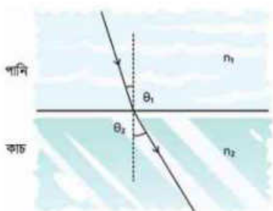
চিত্র 9.05: পানি ও কাচের ভেতর আলোর প্রতিসরণ।
