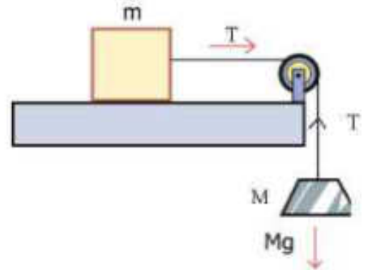
চিত্র 3.09: একটি বস্তুর ভর অন্য বস্তুর উপরে বল প্রয়োগ করছে।
