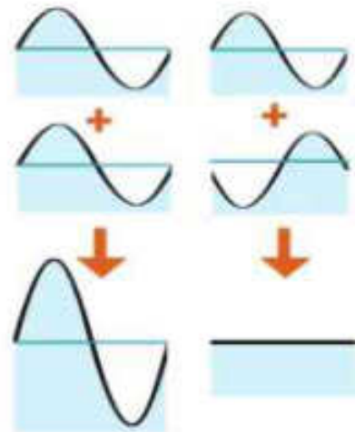
চিত্র 7.03: দুটি তরঙ্গ যোগ হয়ে আরো বড় তরঙ্গ হতে পারে, আবার একটি অন্যটিকে নিরূপক করে দিতে পারে।
