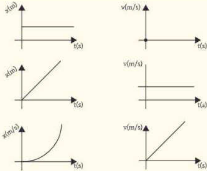
চিত্র 3.01: তিনটি ভিন্ন পরিস্থিতির ক্ষেত্রে অবস্থান-সময় ও বেগ-সময়ের তিন জোড়া প্লটচিত্র।
