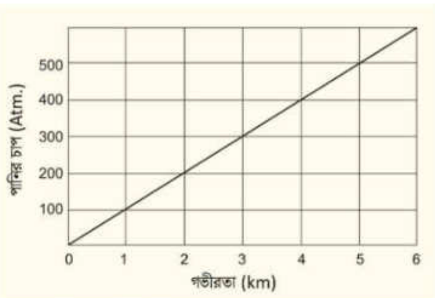
চিত্র ৫.০৩: পানির গভীরতায় সাথে সাথে পানির চাপ বেড়ে যায়।
