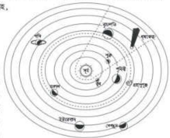
চিত্র ৩.১ : সৌরজগৎ
