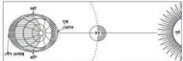
চিত্র ৩.১১ : জোয়ার-ভাটা
